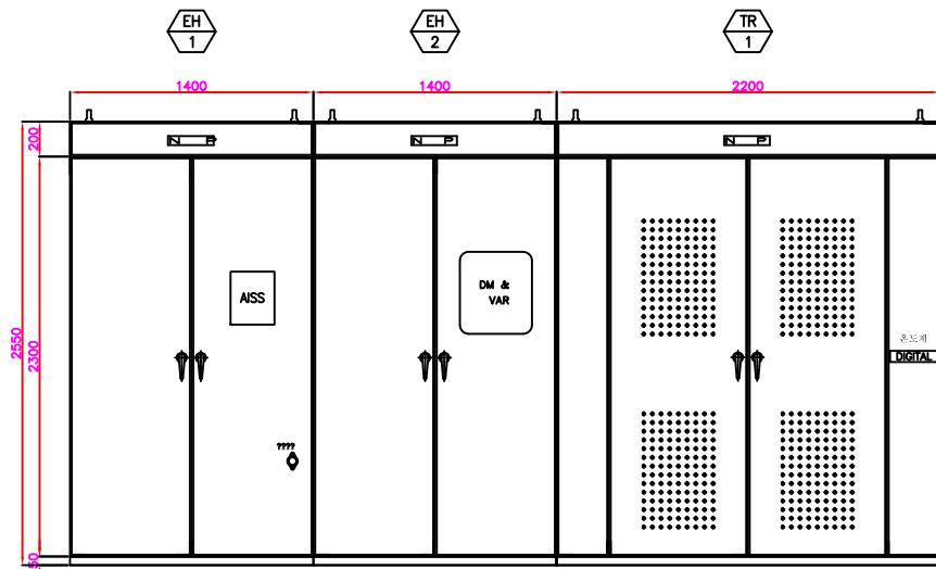
고압반 FRONT VIEW
